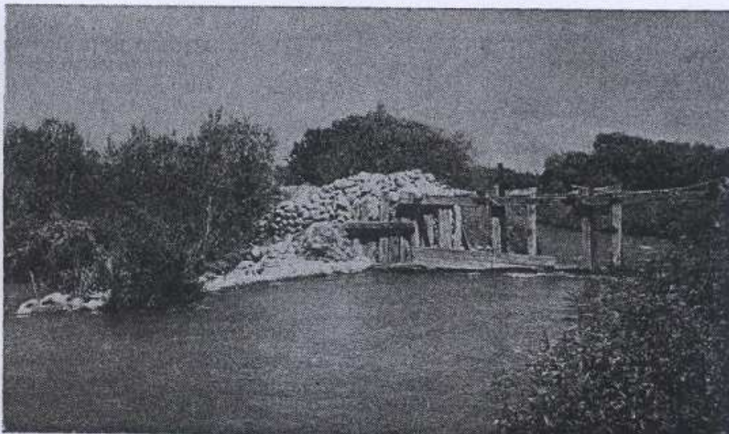
Marco partidor y aparejo de una compuerta rústica en canales de riego de la zona del Plan Chillán.
