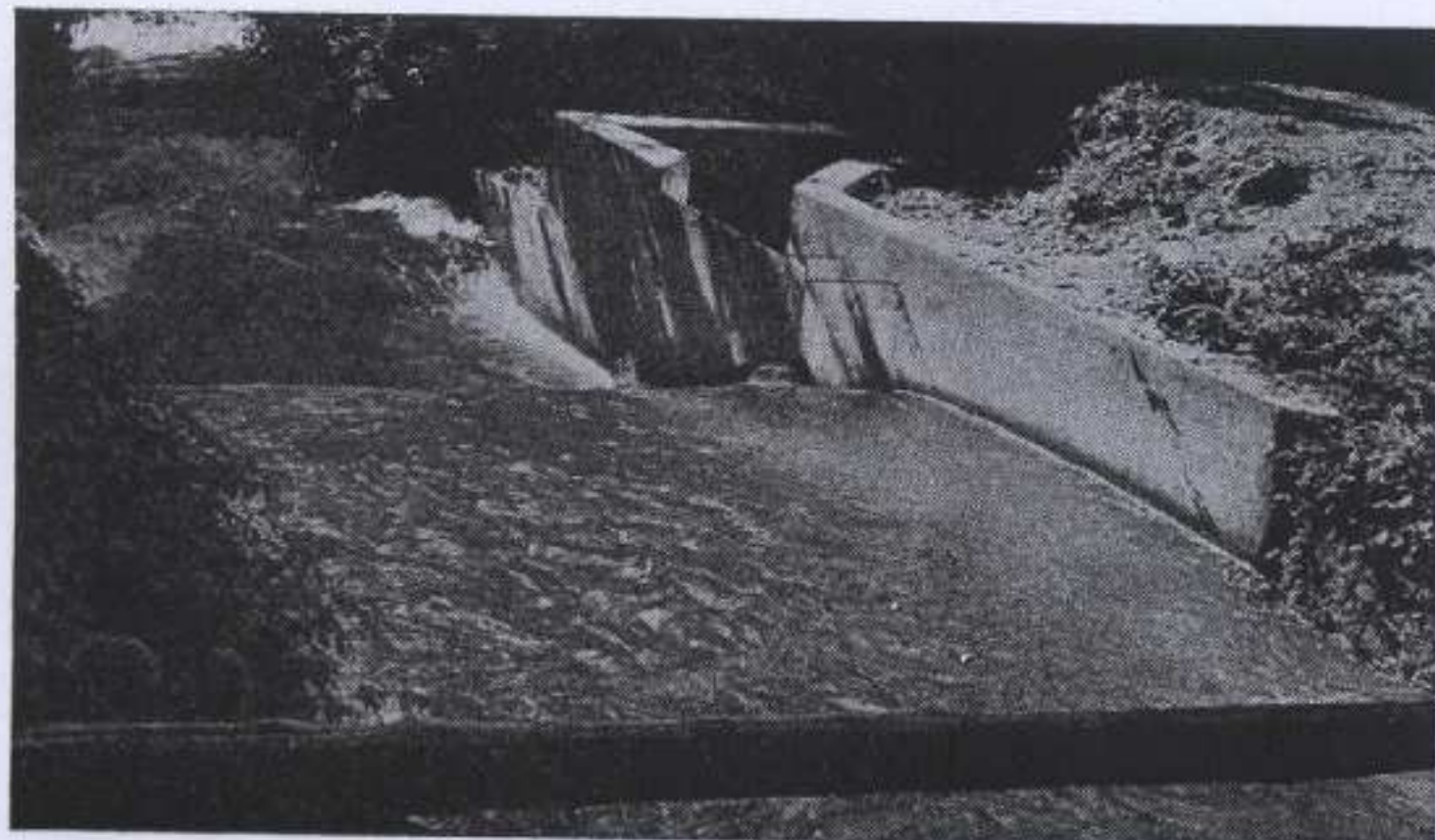
Marco partidor y aparejo de una compuerta rústica en canales de riego de la zona del Plan Chillán.
