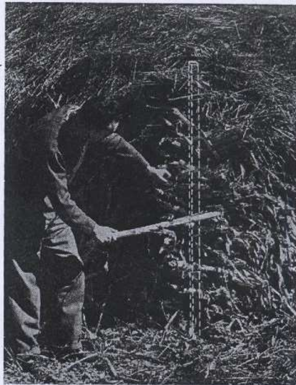
Silo-parva de cañas de maíz que permite apreciar la disposición trabada de las cañas en las esquinas, para dar solidez al silo. Es recomendable estacar el silo como indican las líneas de puntos, para garantizar su estabilidad.
